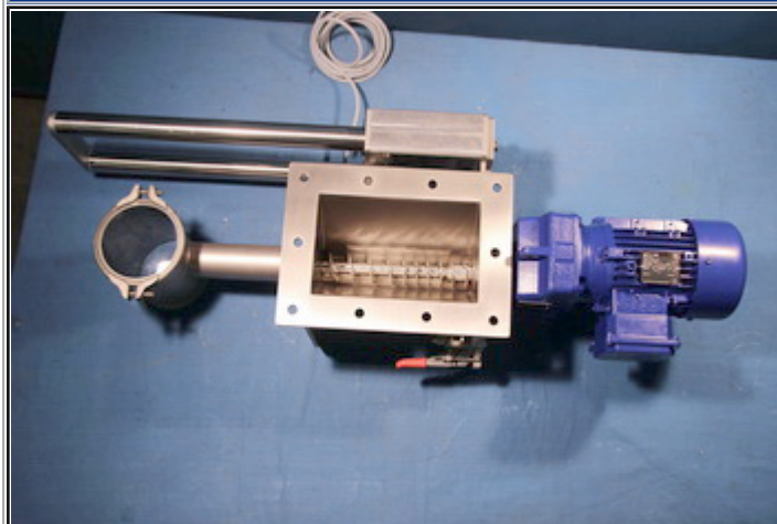
Dosierschnecke mit Gewindeauszugs- und Schwenkvorrichtung
